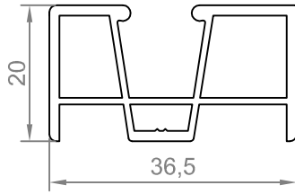
MONTANT PVC
