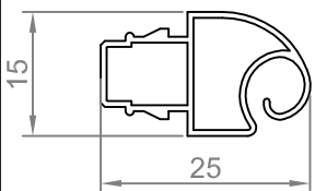
CHARNIERE DE RIVE PVC
