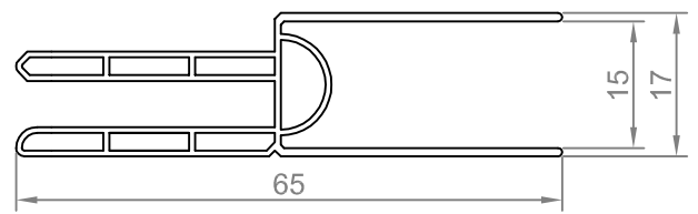
BATTEMENT PVC
